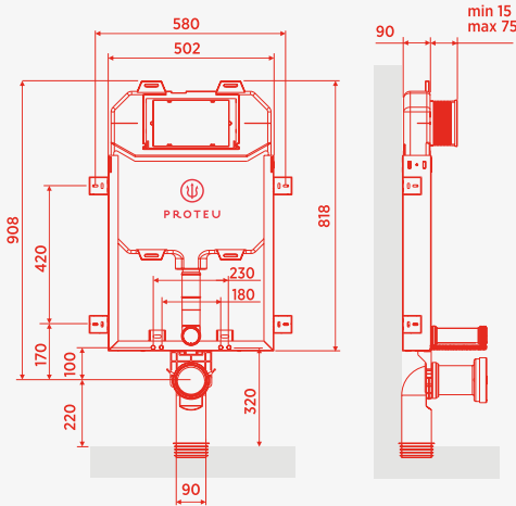
Dimensões
